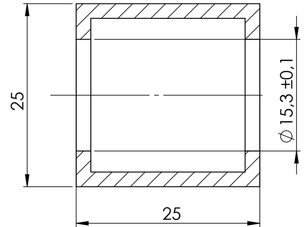
DÉTAIL B ECHELLE 2 : 1
