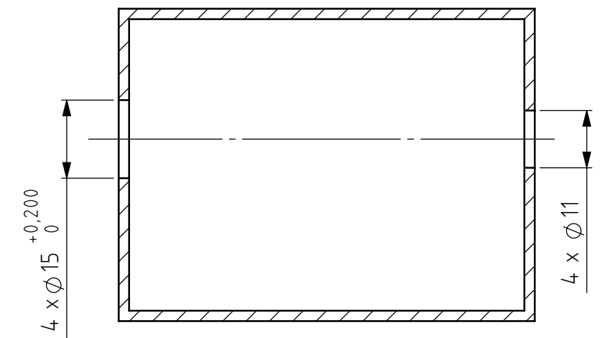
B (1 : 1) fixation des paliers de bras de suspension arrière (x4)
