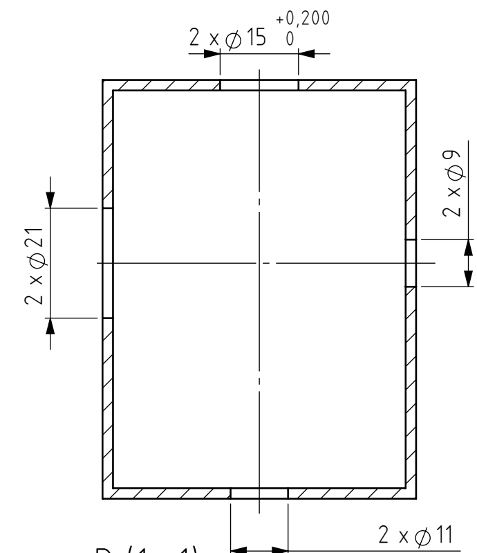
D (1 : 1) fixation de la flasque support moteur (x2)
