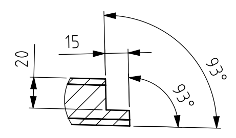
D (2 : 5)
