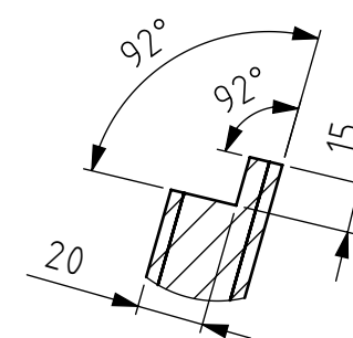
F (2 : 5)
