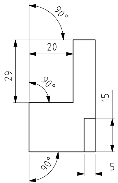
B (1 : 1)
