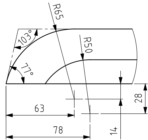
E (1 : 2)
