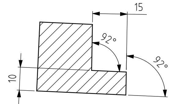
D-D (1 : 1)
