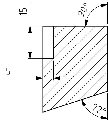
F (1 : 1)
