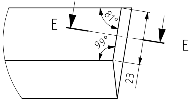
B (1 : 1)
