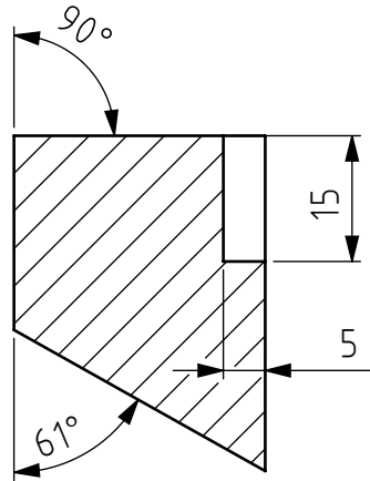
F (1 : 1)
