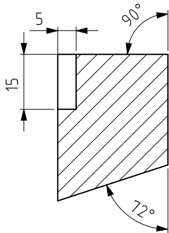
G (1 : 1)
