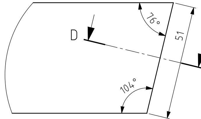
B (1 : 1)
