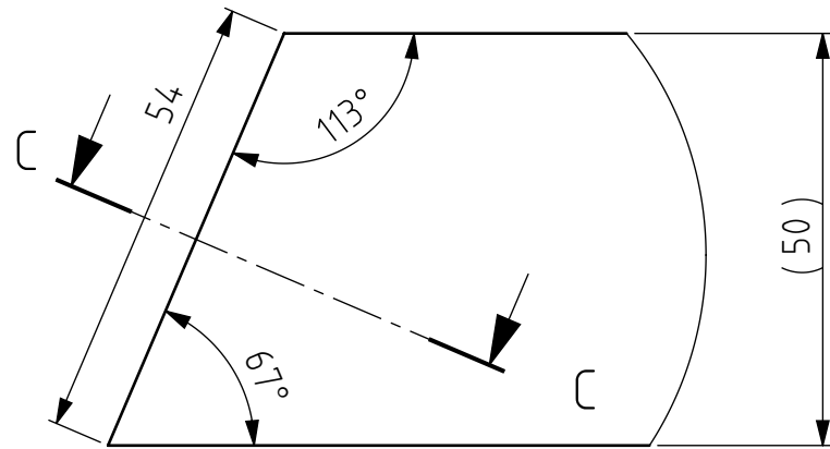
A (1 : 1)
