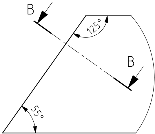
A (1 : 1)
