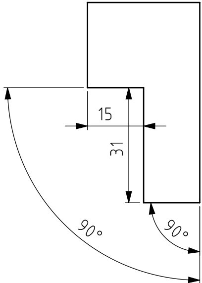
C (1 : 1)
