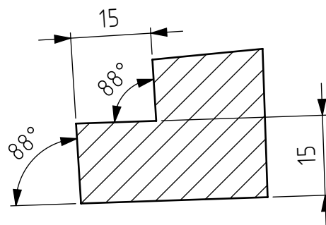
B-B (1 : 1)
