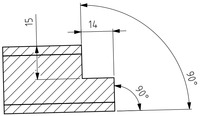
B-B (1 : 1)
