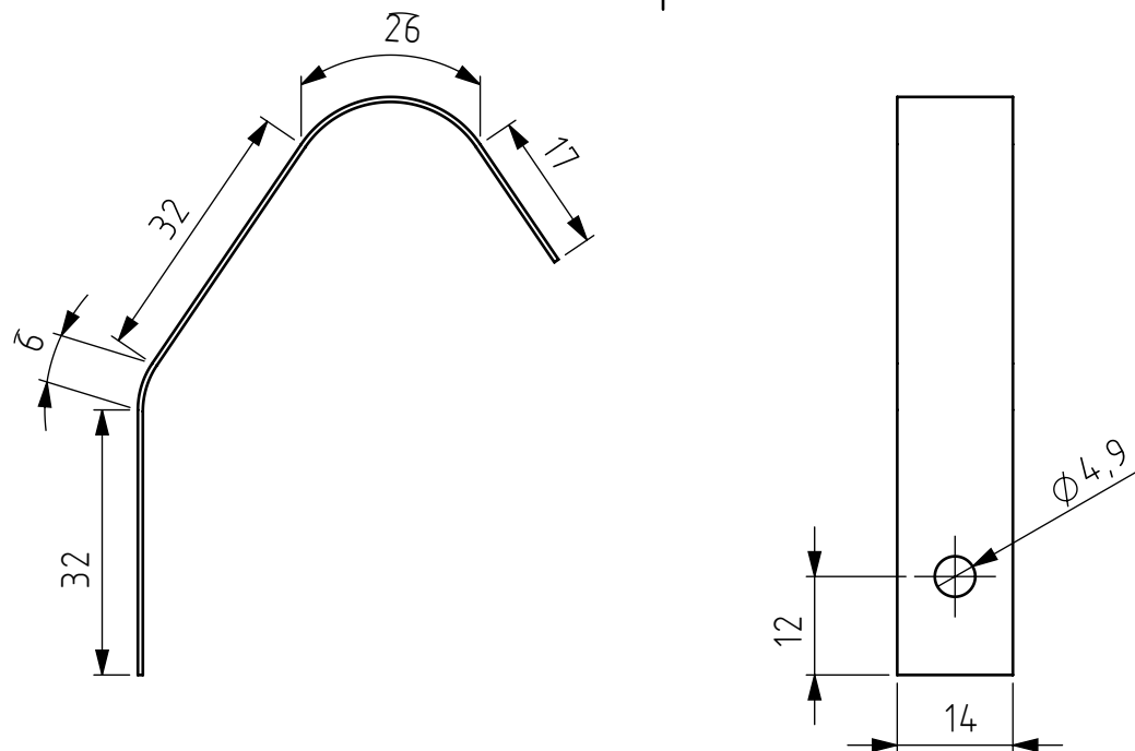
Collier de serrage largeur 14mm, longueur 113mm
